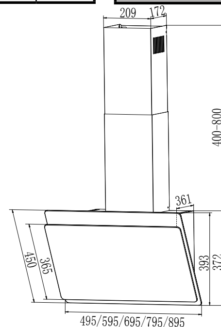
Рис. 1 Внешний вид кухонной вытяжки и схема размеров
