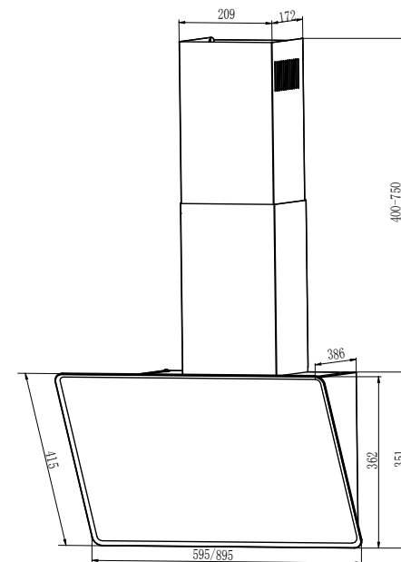
Рис. 1 Внешний вид кухонной вытяжки и схема размеров
