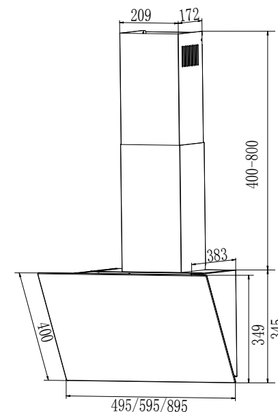
Рис. 1 Внешний вид кухонной вытяжки и схема размеров
