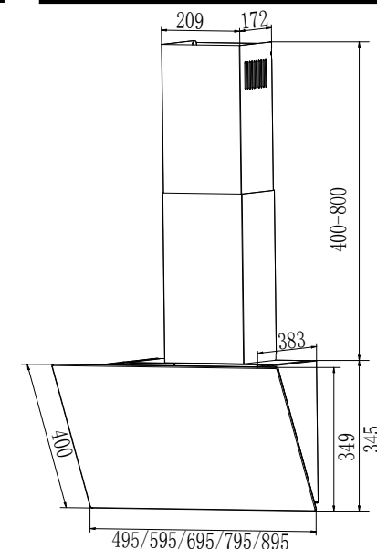
Рис. 1 Внешний вид кухонной вытяжки и схема размеров
